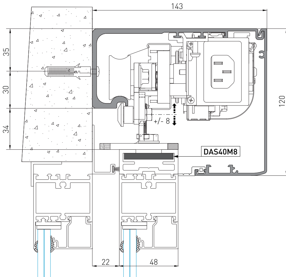
DAS107PLUS-ALU48
